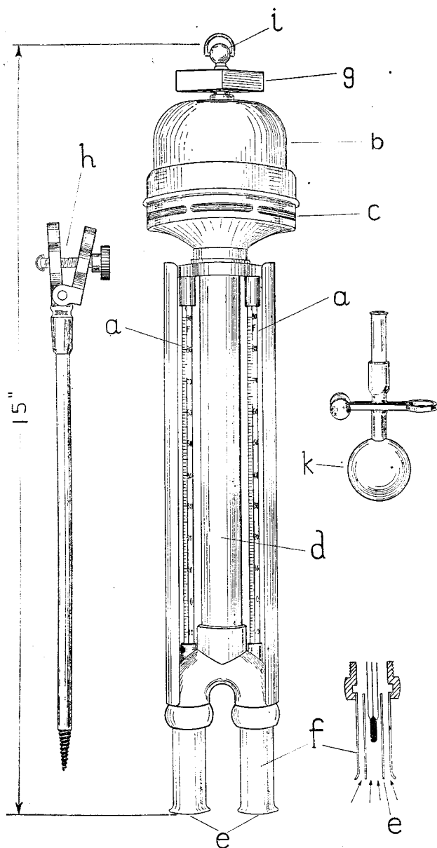
FIG. 15. ASSMANN PSYCHROMETER
