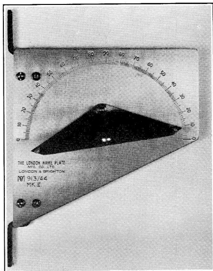
METEOROLOGICAL OFFICE ALIDADE, MK. II
