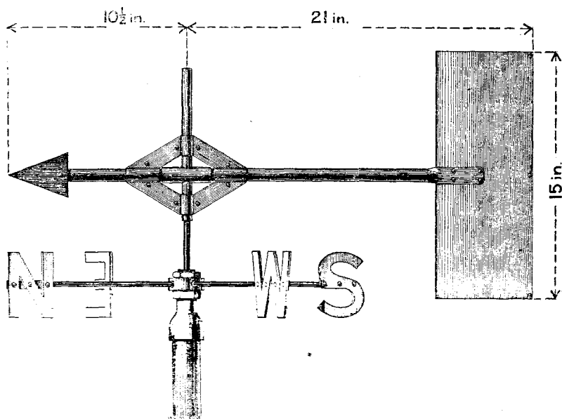
FIG. 16. WIND VANE
