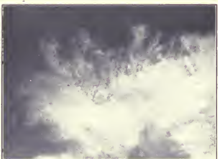
Fig. 29. Fibrous cirrus.
