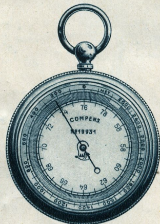
N° 210 Altimètre de poche de haute précision, type Standard, mouvement très soigneusement réglé et compensé, boîtier doré, nickelé ou chromé en forme montre, cadrans argentés et gravés, échelle des hauteurs mobile.
