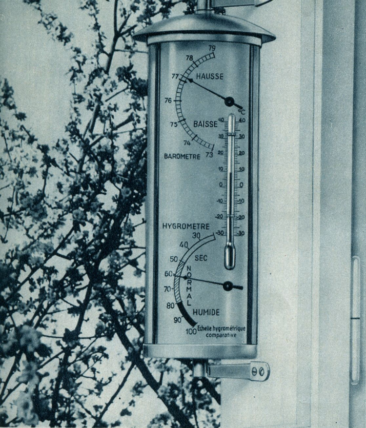
No 705 «MÉTÉOREX» Cette combinaison d'instruments pour la prévision du temps et pour l'observation des conditions climatiques à l'extérieur est construite en particulier pour être montée aux fenêtres, balcons etc.; elle permet une lecture facile de l'intérieur.
