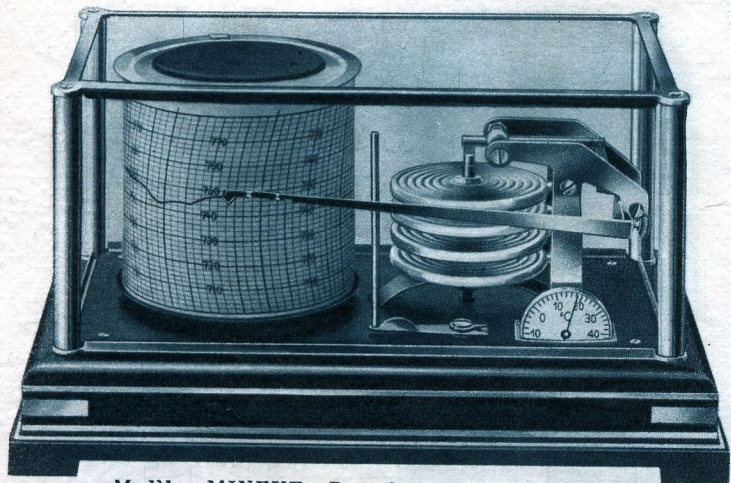
Modèle « MINEUF », Baromètre enregistreur à la portée de tout le monde. Instrument de toute première qualité. Mouvement d'horlogerie de 8 jours, cage chromée avec socle en métal chromé et laqué noir, avec accessoires.
