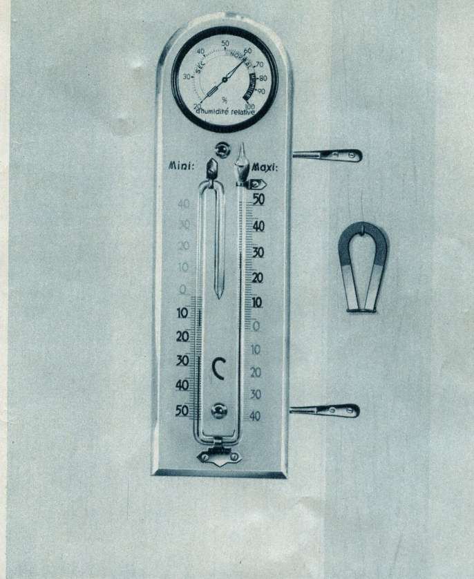
No 719H Thermomètre minima-maxima sur cadran opale de 28×8 cm, combiné avec un hygromètre à cheveux (mesureur d'humidité), diamètre du cadran 60 mm.
