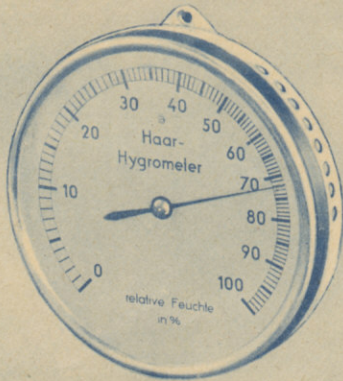
Präzisions-Haarhygrometer in Metallgehäuse, Skala 100 mm Ø Nr. 111
