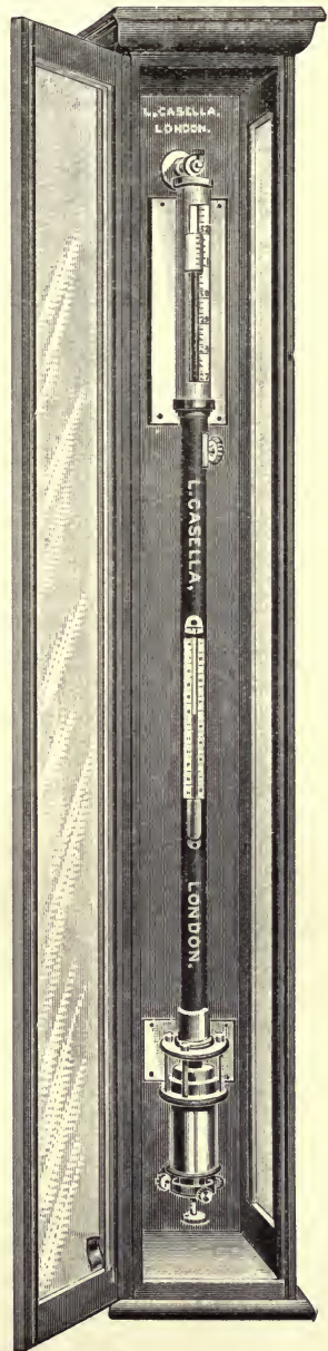
FIG. 23.—FORTIN BAROMETER.
