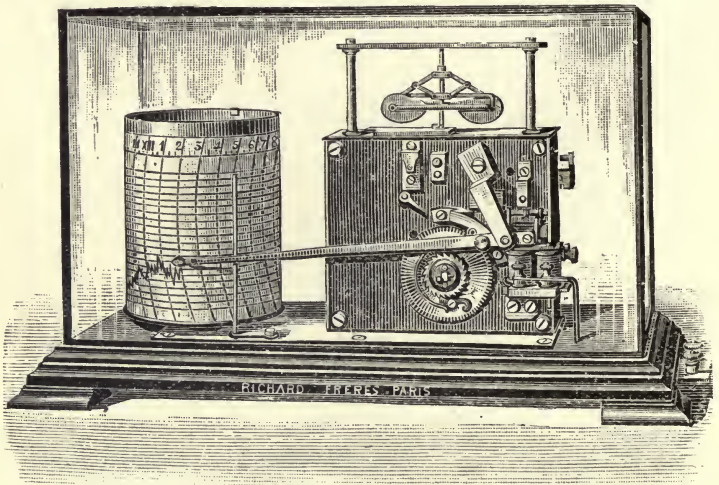
FIG. 83.—RICHARD'S ANÉMO-CINÉMOGRAPHE (Second Form).
