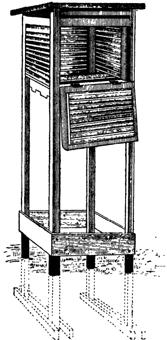
Fig. 1.—Stevenson Screen.
