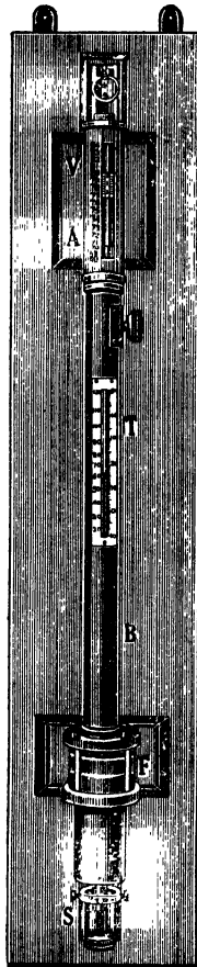
Fig. 4(a).—Fortin's barometer.
